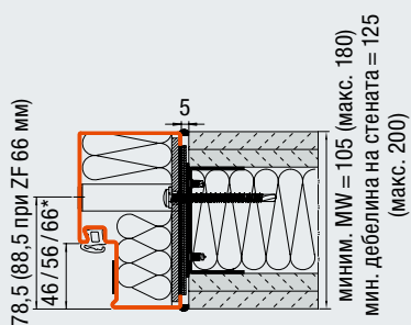
Блок-каса със съосни капачки и скрит монтаж с дюбели – в отвора (Преградна стена)
