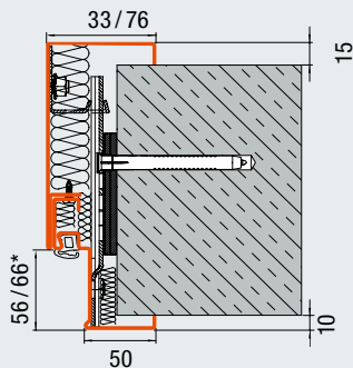
Обхващаща каса от 2 части със скрит монтаж с дюбели и пълнеж от минерална вата (Зид / Гладка лицева стена / Бетон, също и за измазан зид)
