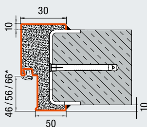
Обхващаща каса с монтаж чрез заваряване (Газобетон)
