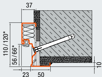
Каса DryFix с диагонално фиксиране (Измазан зид)
