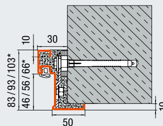
Ъглова каса със скрит монтаж с дюбели (Гладка лицева стена / Бетон)
