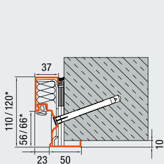
Каса DryFix с диагонално фиксиране (Гладка лицева стена / Бетон)
