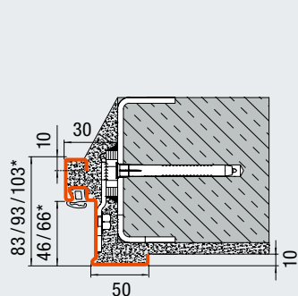
Ъглова каса с монтаж чрез заваряване (Газобетон)
