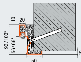
Ъглова каса с диагонално фиксиране (Зид / Гладка лицева стена / Бетон)
