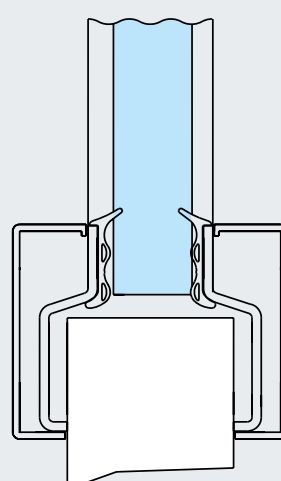
Алуминиев покриващ профил
