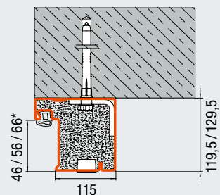
Блок-каса със съосни капачки и скрит монтаж с дюбели - пред отвора (Зид / макс. врати Т30)
